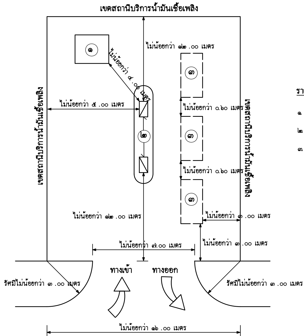
ตัวอย่างภาพประกอบที่ ๓ สถานบริการน้ำมันเชื้อเพลิงที่มีทางเข้าและทางออกสำหรับยานพาหนะทางเดียว
